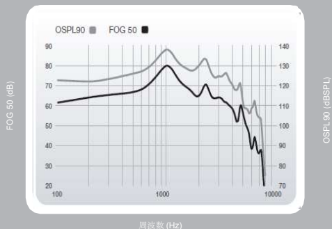
BTE 13 パワープラス (標準チューブ)
