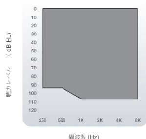
Muse iQ BTE 13 適応聴力範囲
