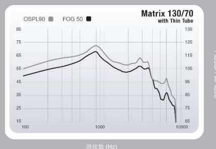
Muse iQ BTE 13 (スマートイヤチューブ)
